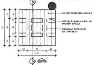
05 PLANTA BAIXA - DETALHE 05 escala 1:30
