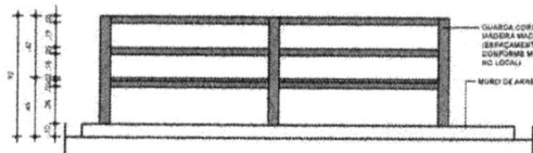
02 V02 - DETALHE 01 escala 1:20
