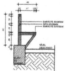
04 CORTE AA - DETALHE 01 escala 1:20
