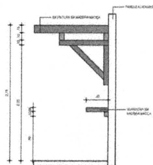
03 CORTE AA - DETALHE D7 escala 1:20
