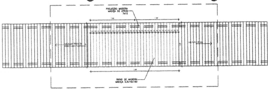
01 PLANTA BAIXA - DETALHE 08 escala 1:20
