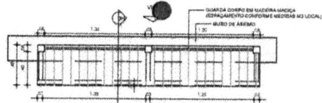
01 DETALHE 01 - BANCO escala 1:20
