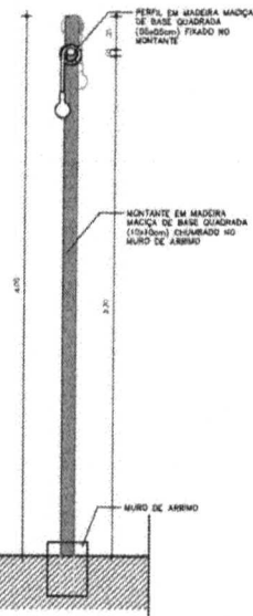
08 V02 - DETALHE 02 escala 1:20
