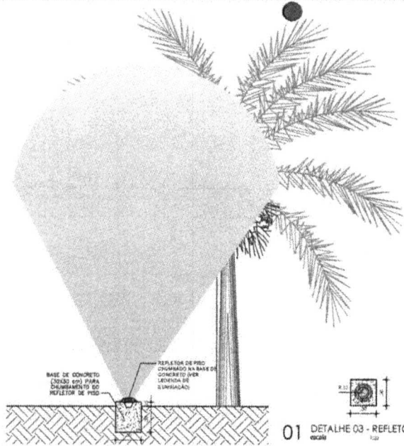
02 CORTE AA - DETALHE 03 escala 1:20
