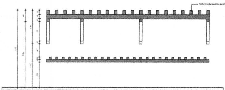
02 VISTA D1 - DETALHE D7 escala 1:20
