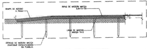
02 VISTA 01 - DETALHE 08 escala 1:20
